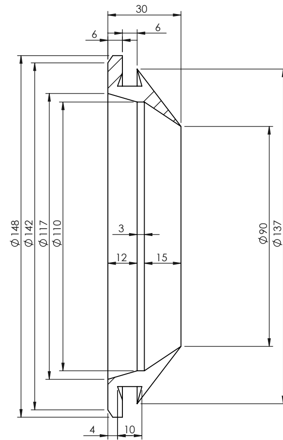
SEZIONE A-A SCALA 1:1.5
